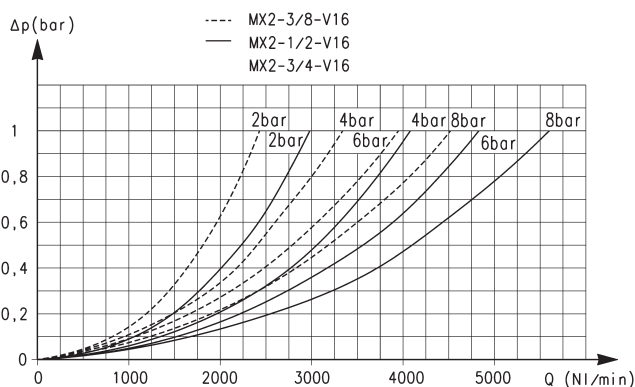
Діаграми для клапанів з електропневматич або пневматичним керуванням МХ2
