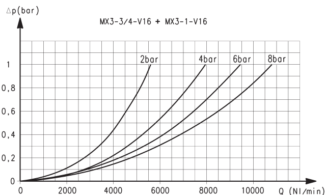
Діаграми для клапанів з електропневматич або пневматичним керуванням МХ3
