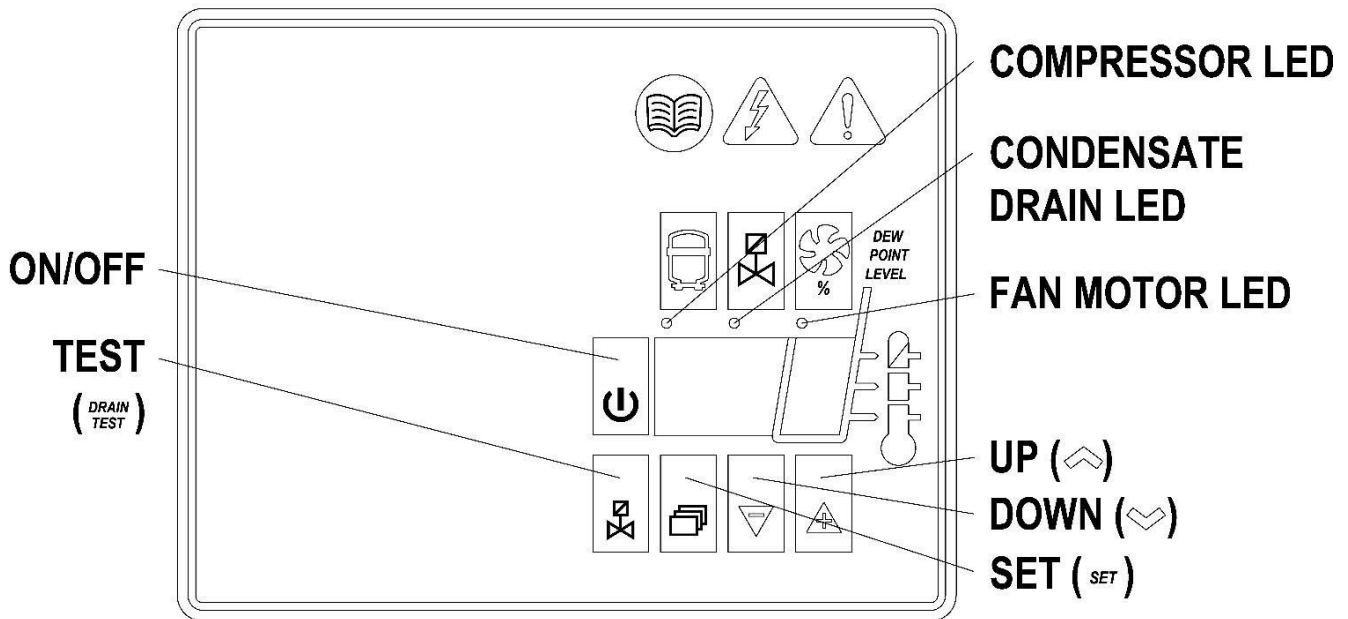
Візуалізація дисплея та світлодіодні індикатори (DD36 ÷ DD1000)
